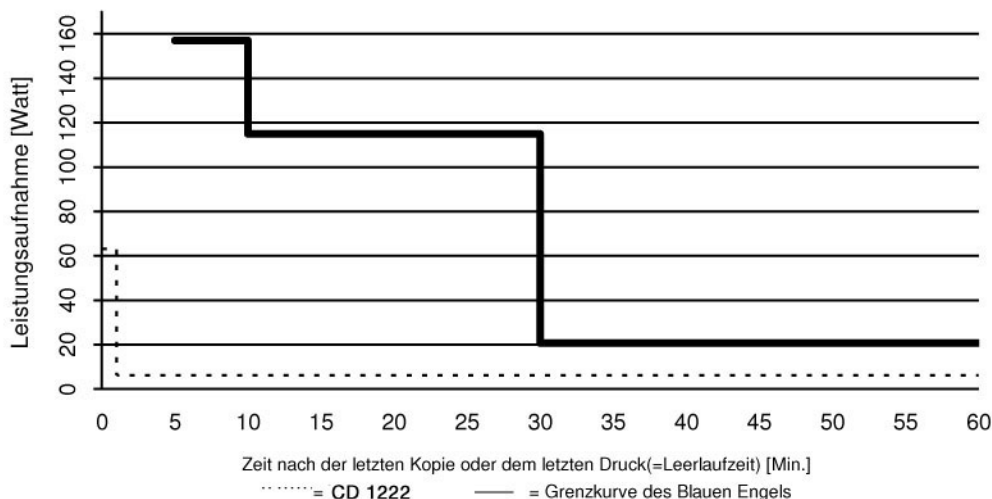
Leistungsaufnahme und Aktivierungszeit des CD 1222 in der Zeit nach dem letzten Druck
